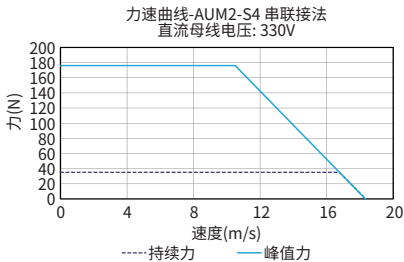
■ 力-速度 曲线
