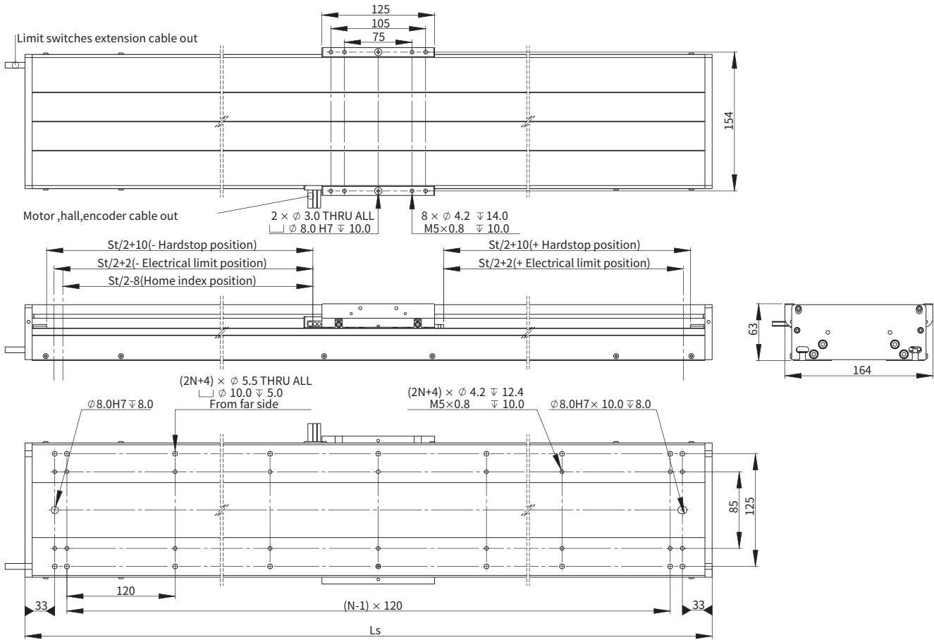
■ DGL150-AUM2-S4 尺寸图
