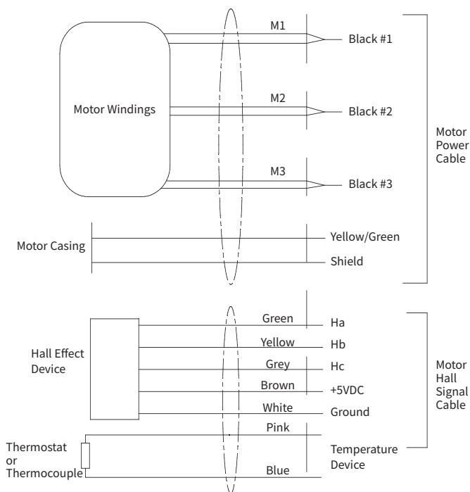
电缆连接信息 (600Vdc)
