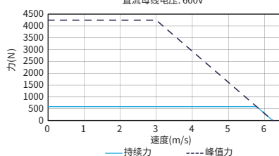
力速曲线-AUM5-S6 串联接法 直流母线电压: 600V
