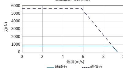
力速曲线-AUM5-S8-V107 串联接法 直流母线电压: 600V
