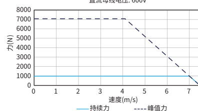
力速曲线-AUM5-S10-V107 串联接法 直流母线电压: 600V
